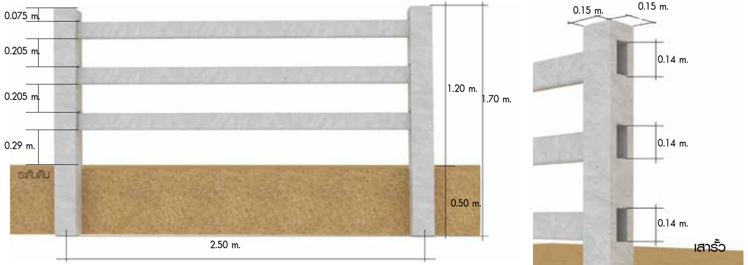
รั้วคานบอย พีซีซี ทางเลือกใหม่สำหรับงานรั้ว ติดตั้งง่าย ได้มาตรฐาน แข็งแรงทนทาน และสวยงาม
